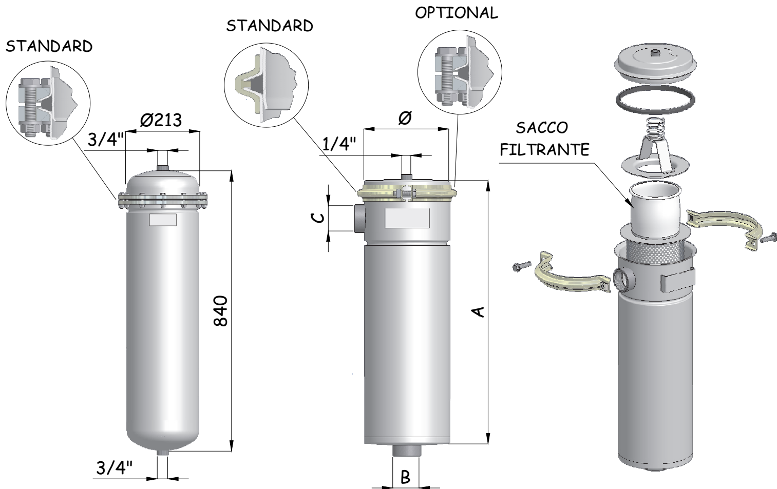
PREFILTRO A SACCO Ø213 Cod. 8.0584.0
